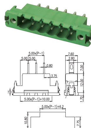
P/N: BC5EHDKM-XX-P XX= N° CONTACTS
