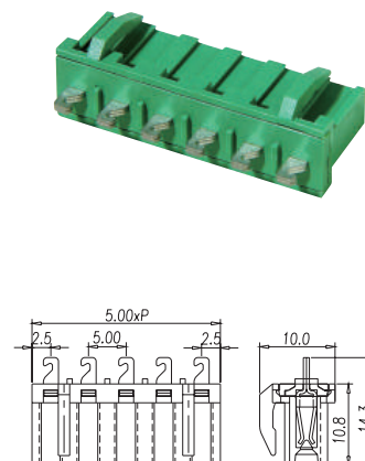
P/N: BC5ESDN-XX-P XX= N° CONTACTS
