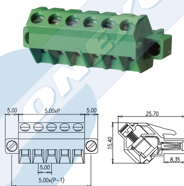
P/N: BC5ESDAM-XX-P XX= N° CONTACTS
