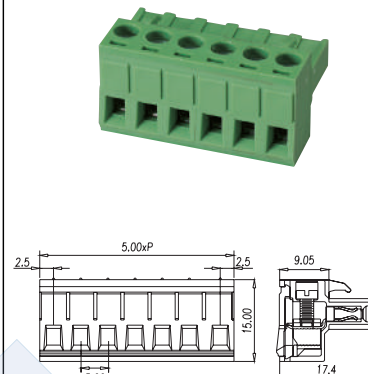
P/N: BC5ESDT-XX-P XX= N° CONTACTS
