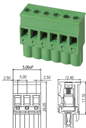
P/N: BC5ESDPL-XX-P XX= N° CONTACTS
