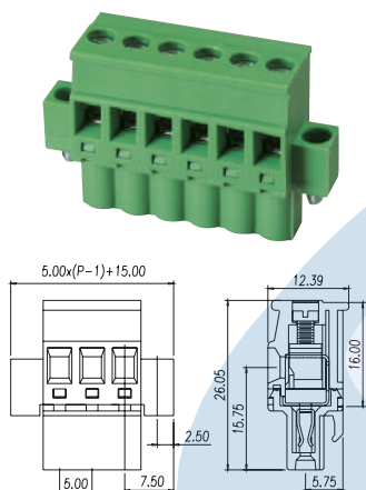
P/N: BC5ESDPLM-XX-P XX= N° CONTACTS
