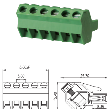
P/N: BC5ESDA-XX-P XX= N° CONTACTS
