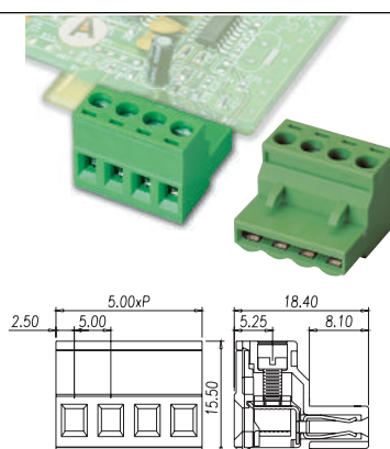
* 12 A IEC / 250 V IEC P/N: BC5ESDG-XX-P XX= N° CONTACTS
