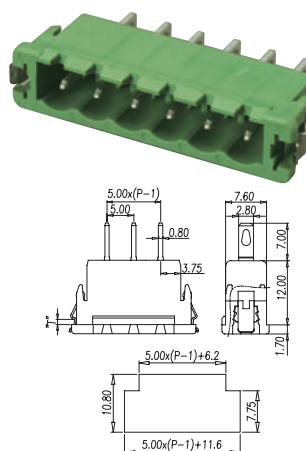
P/N: BC5EHDK-XX-P XX= N° CONTACTS
