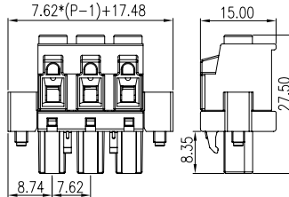
P/N: BC3ESNP-XX-P XX= N° CONTACTS
