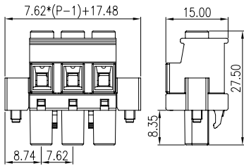
P/N: BC3ESNP-XX-P XX= N° CONTACTS
