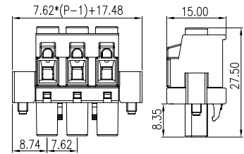
P/N: BC3ESNP-XX-P XX= N° CONTACTS
