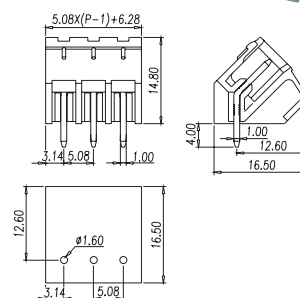
P/N: BC2EHDAC-XX-P XX= N° CONTACTS
