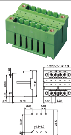
P/N: BC2EHDBVM-XX-P XX= N° CONTACTS
