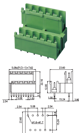
P/N: BC2EEHDV-XX-P XX= N° CONTACTS
