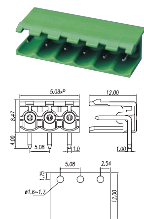
P/N: BC2EHDR-XX-P
