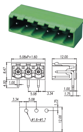
P/N: BC2EHDRC-XX-P
