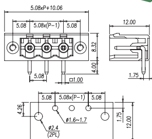
P/N: BC2EHDRM-XX-PEVER XX= N° CONTACTS
