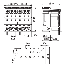
P/N: BC2EHDBR-XX-P XX= N° CONTACTS
