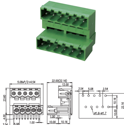
P/N: BC2EEHDC-XX-P XX= N° CONTACTS
