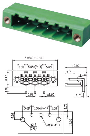
P/N: BC2EHD RM-XX-P
