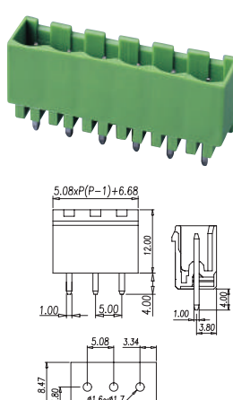
P/N: BC2EHDVC-XX-P
