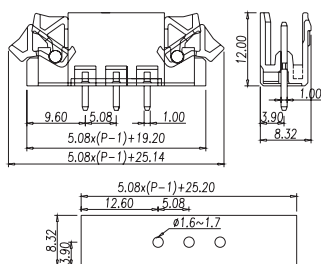
P/N: BC2EHDVL-XX-P XX= N° CONTACTS
