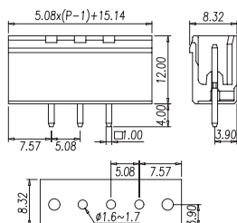
P/N: BC2EHDVM-XX-PEVER XX= N° CONTACTS
