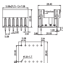
P/N: BC2EHDBV-XX-P XX= N° CONTACTS
