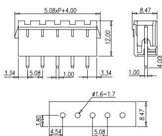
P/N: BC2EHDVT-XX-P XX= N° CONTACTS
