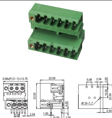
P/N: BC2EEHDRML-XX-P XX= N° CONTACTS
