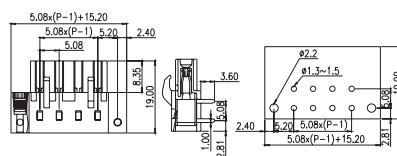
*12 A IEC P/N: BC2ESDCRM-XX-P XX= N° CONTACTS
