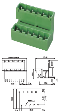
P/N: BC2EEHDVC-XX-P XX= N° CONTACTS
