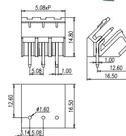
P/N: BC2EHDA-XX-P XX= N° CONTACTS
