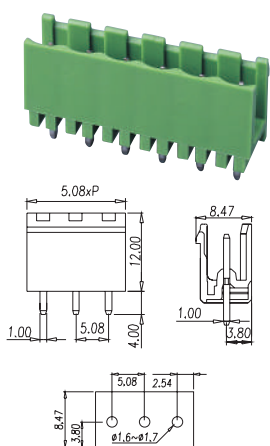
P/N: BC2EHDV-XX-P
