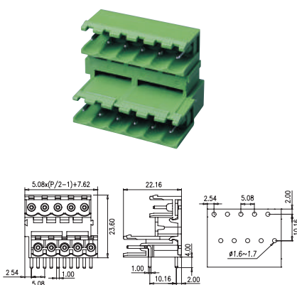
P/N: BC2EEHDR-XX-P XX= N° CONTACTS
