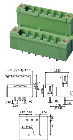
P/N: BC2EEHDVM-XX-P XX= N° CONTACTS
