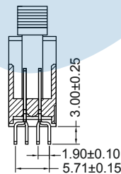
SEC. A-A
