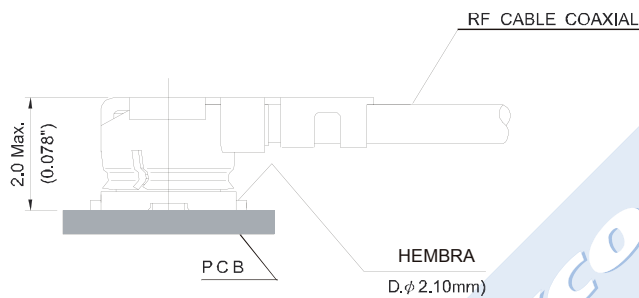
Conector 2704 con 2702
